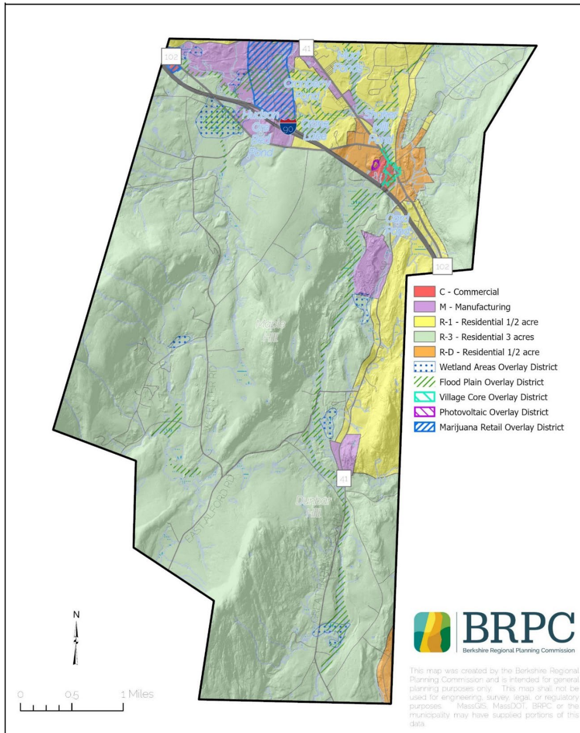
Fig. 3.5. Zoning
