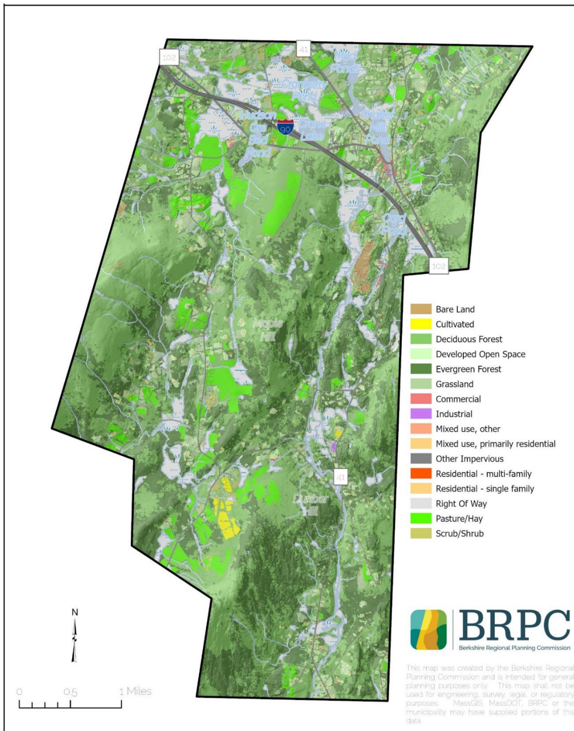
Fig. 3.3. Land Use
