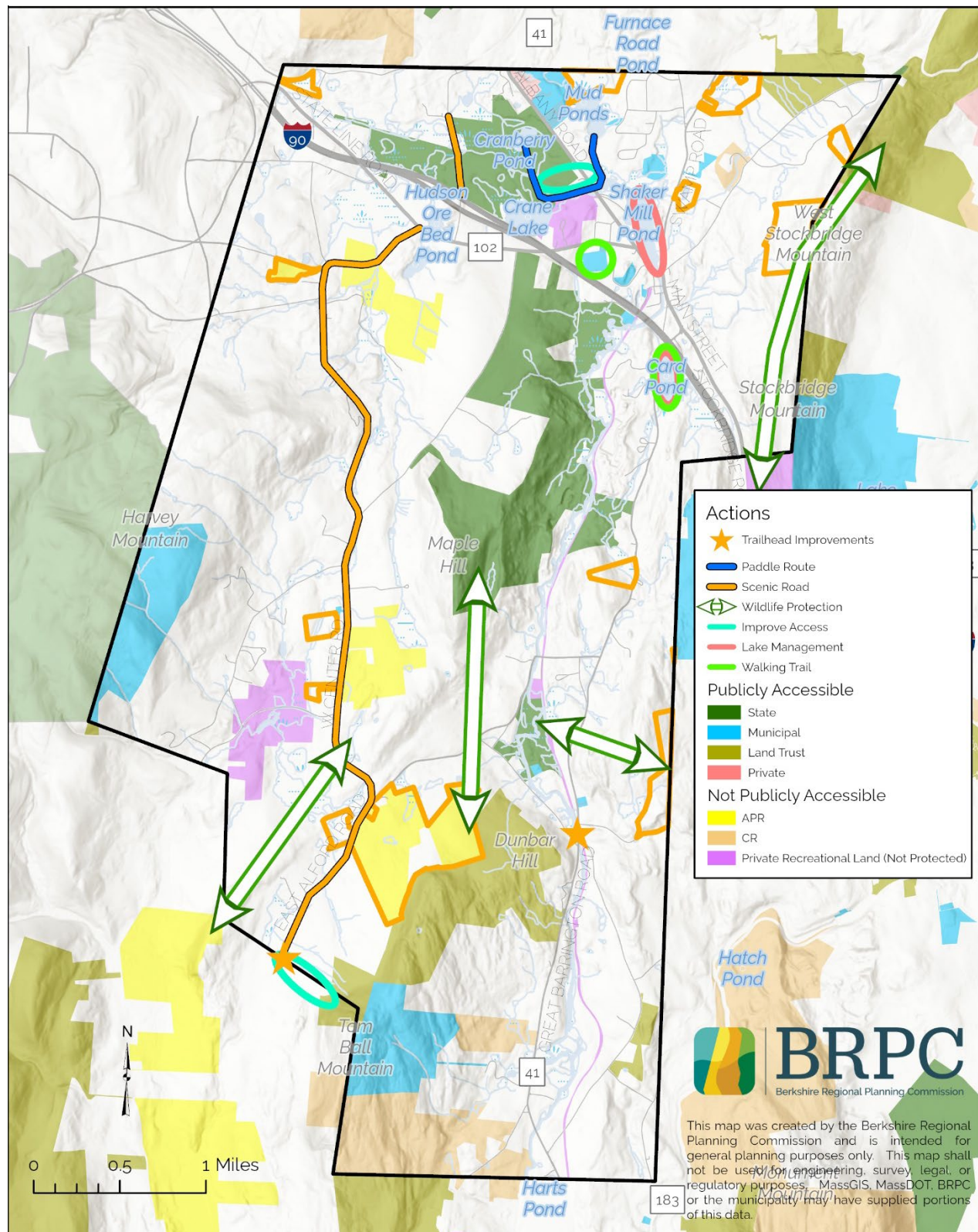
Fig. 7.5. Action Map
