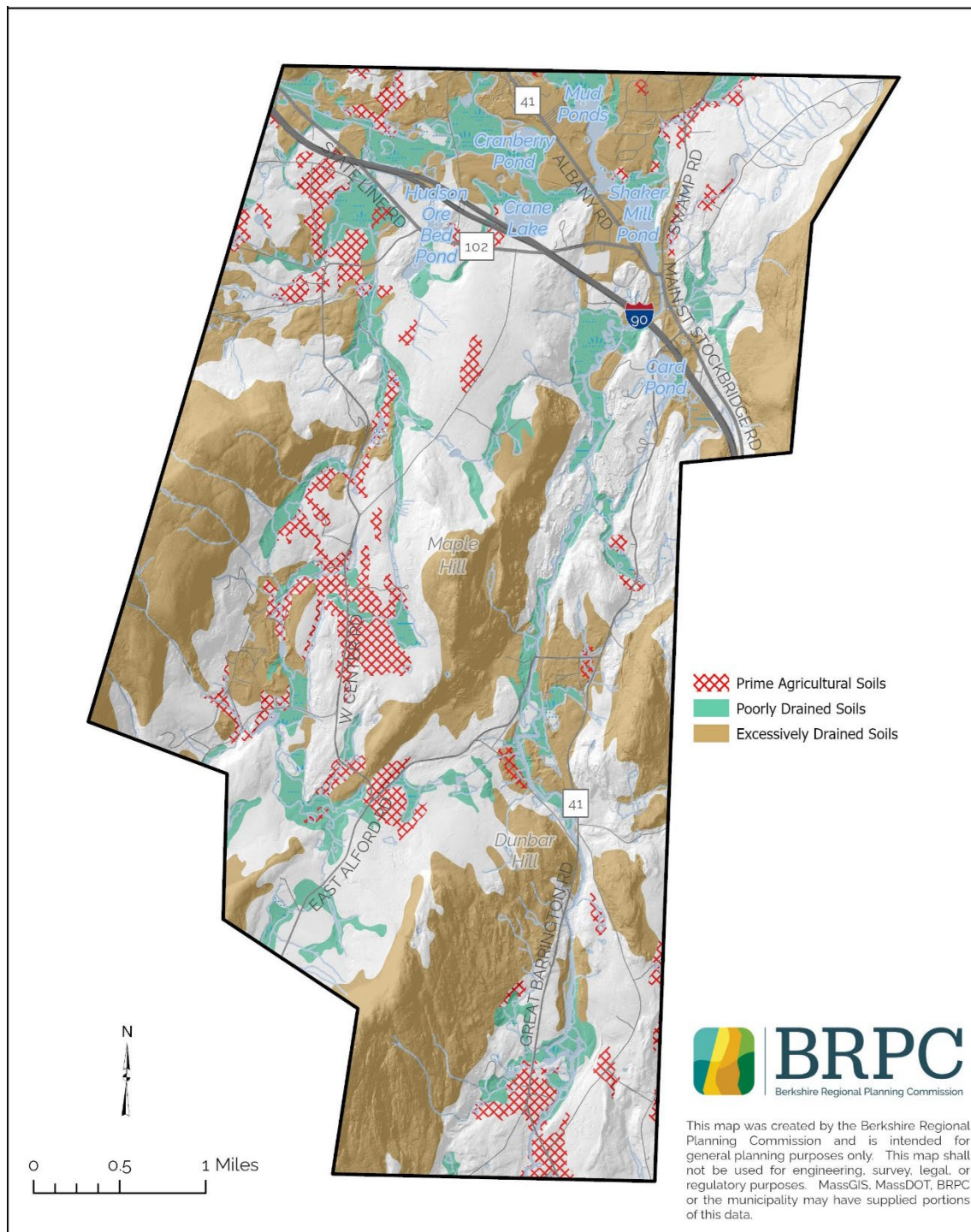
Fig. 4.2. Soils
